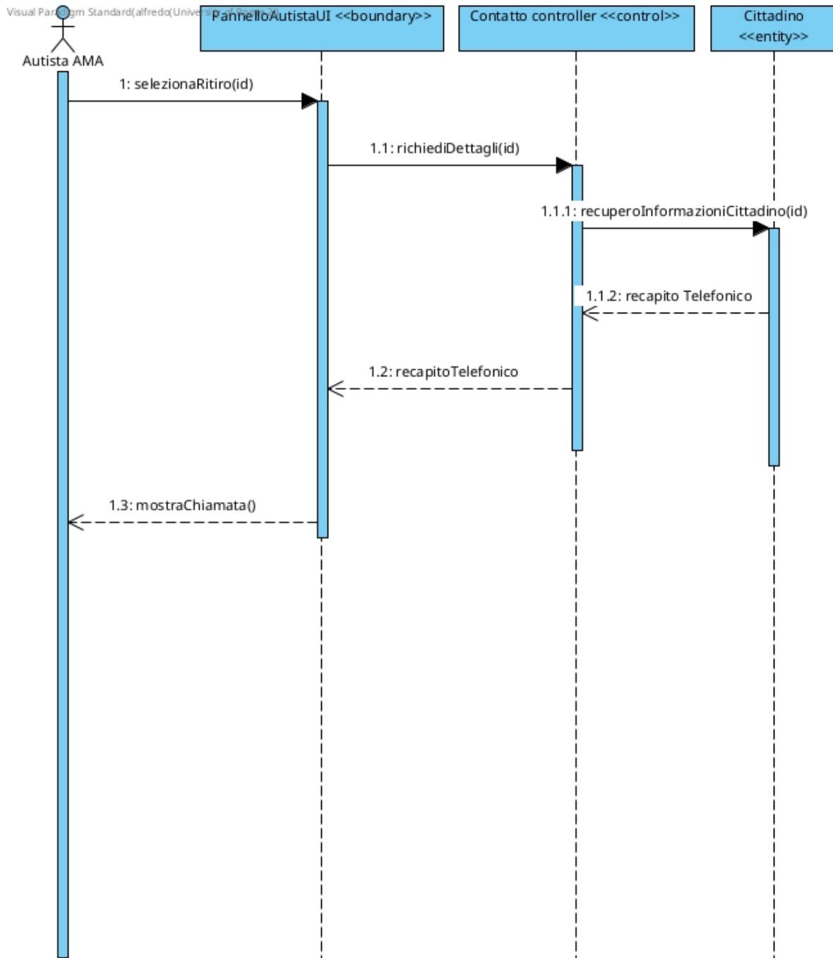
Figura 33: Sequence Diagram — Chiamare cittadino
