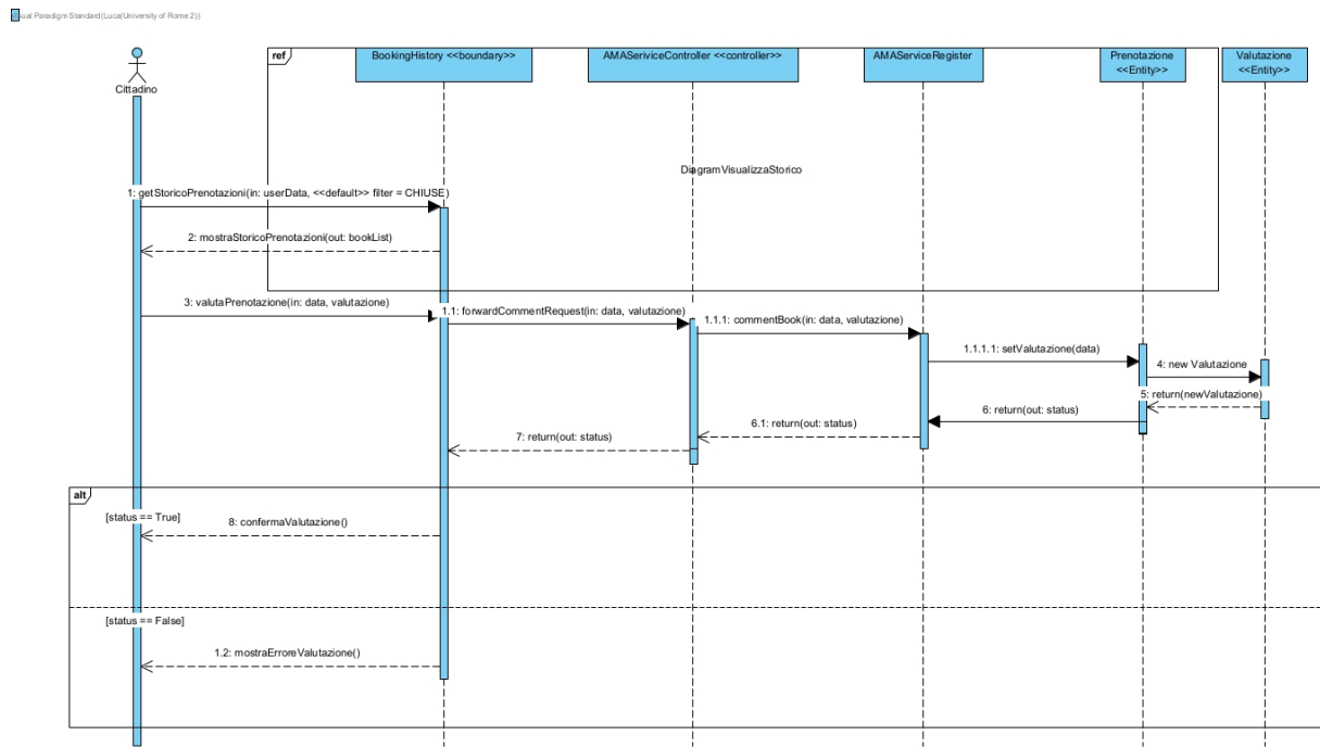
Figura 30: Sequence Diagram — Valutare il servizio
