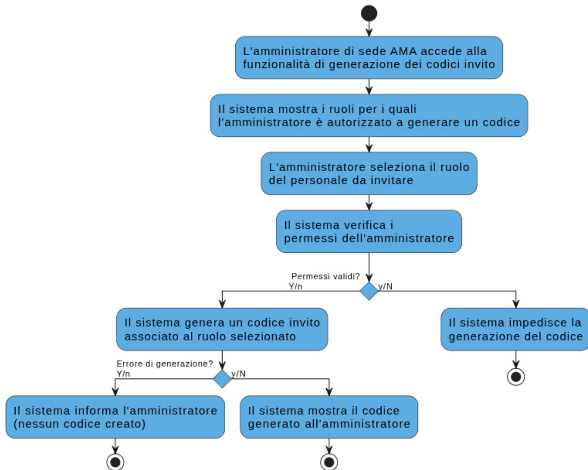
Figura 18: Activity Diagram — Generare codice di invito (Amministratore Sede)
