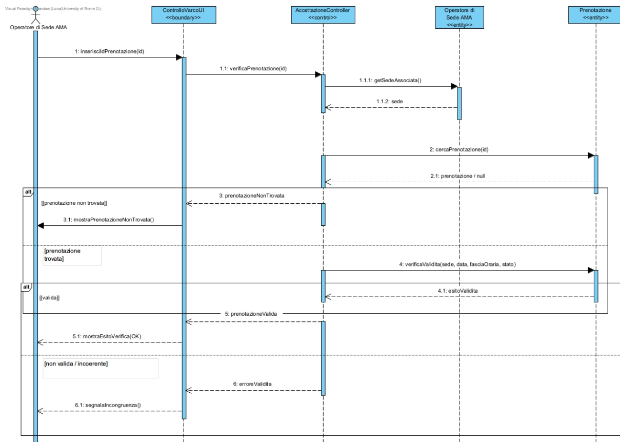
Figura 35: Sequence Diagram — Verificare prenotazione del cittadino
